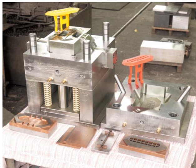
「側溝100」の特注金型
